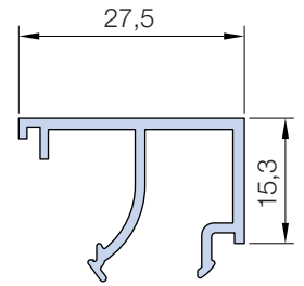
PL 1128 264 g/m
