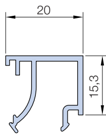
PL 1120 235 g/m
