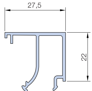
PL 1428 312 g/m
