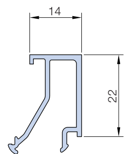
PL 1414 257 g/m
