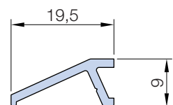
PL 20100 129 g/m
