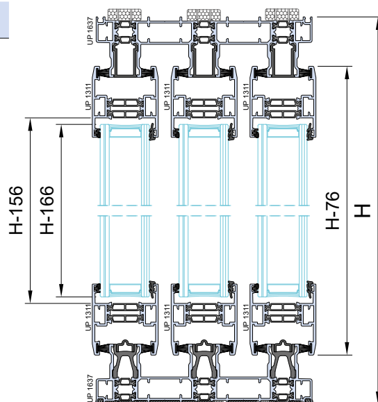
Sez. A-A
