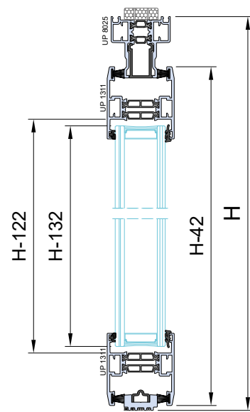
Sez. A-A
