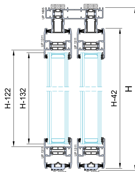
Sez. A-A
