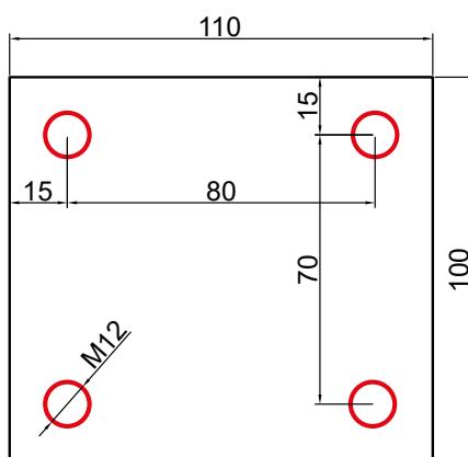
Dimensioni della piastra di fissaggio per soluzione monovia (spessore 10mm)
