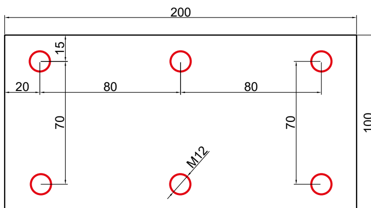
Dimensioni della piastra di fissaggio per soluzione a due vie (spessore 10mm)
