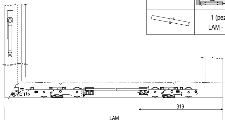
Formule di taglio asta di giunzione ACP 90212
