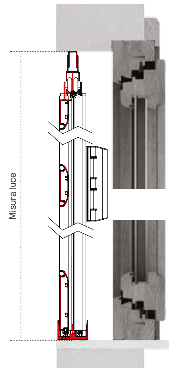
SEZ. VERTICALE
