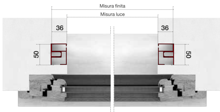
SEZ. ORIZZONTALE
