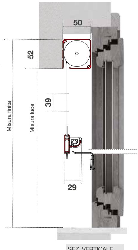
SEZ. VERTICALE
