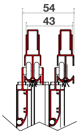
DETTAGLIO DOPPIO BINARIO SUPERIORE (OPTIONAL) PER 3 ANTE IMPACCHETTATE SU UN LATO.
