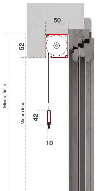
SEZ. VERTICALE
