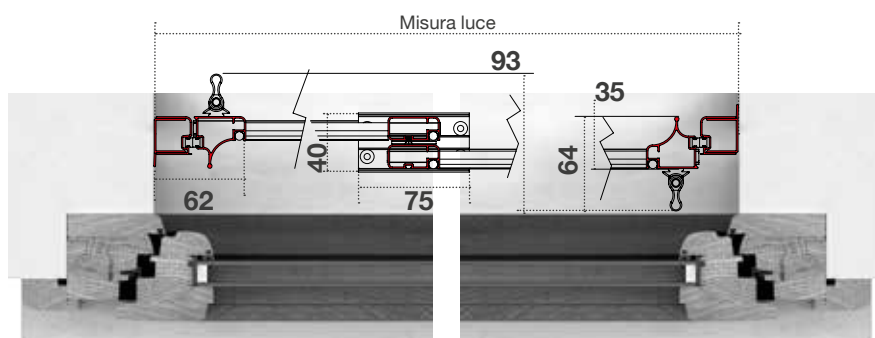
SEZ. ORIZZONTALE
