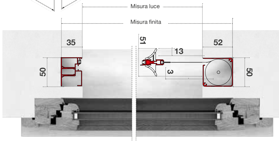
SEZ. ORIZZONTALE
