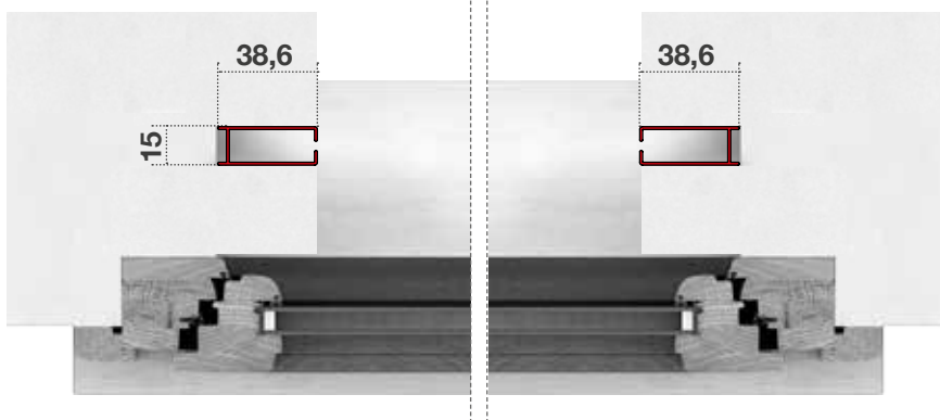
SEZ. ORIZZONTALE
