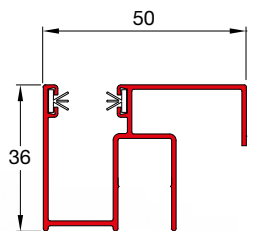
STANDARD GUIDA MODELLO 02
