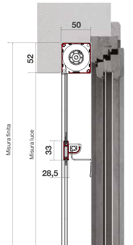
SEZ. VERTICALE
