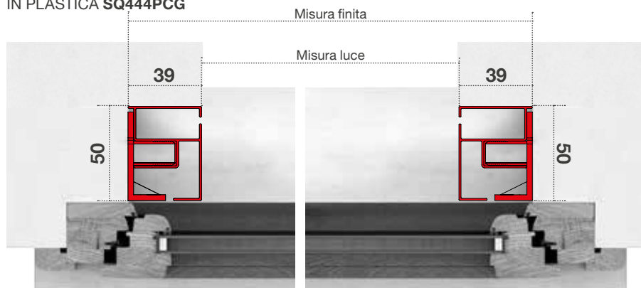
SEZ. ORIZZONTALE
