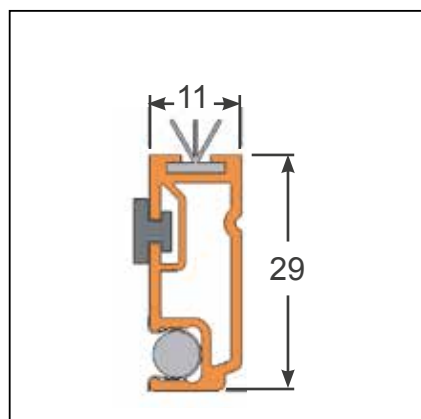
Sezione profilo con spazzolino e magnete (optional).
