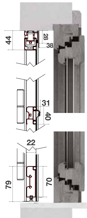
SEZ. VERTICALE
