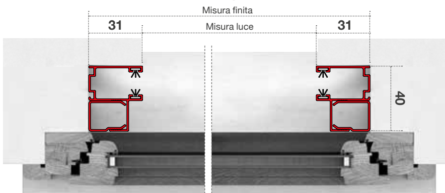
SEZ. ORIZZONTALE
