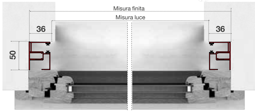
SEZ. ORIZZONTALE
