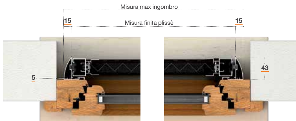
SEZ. ORIZZONTALE
