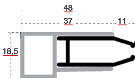
GUIDA STANDARD
