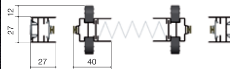
SEZ. ORIZ. GIOCONDA REVERSIBILE
