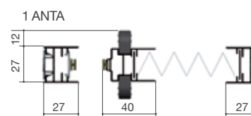
SEZ. ORIZZONTALE GIOCONDA LATERALE
