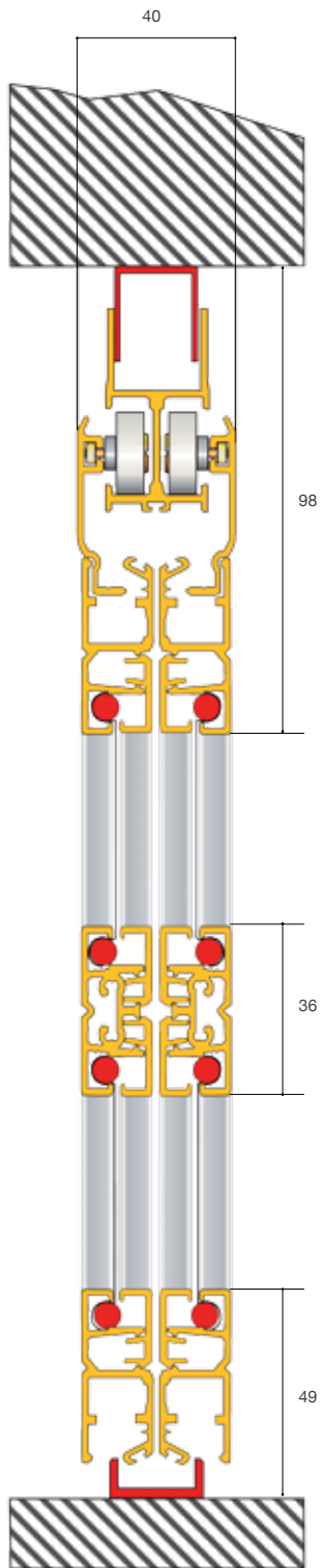
SEZ. VERTICALE
