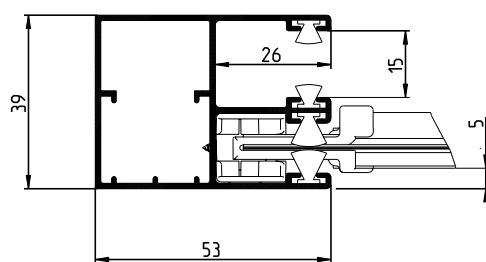
SEZIONE GUIDA
