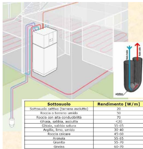
Pompa di calore terra/acqua a sonda verticale
