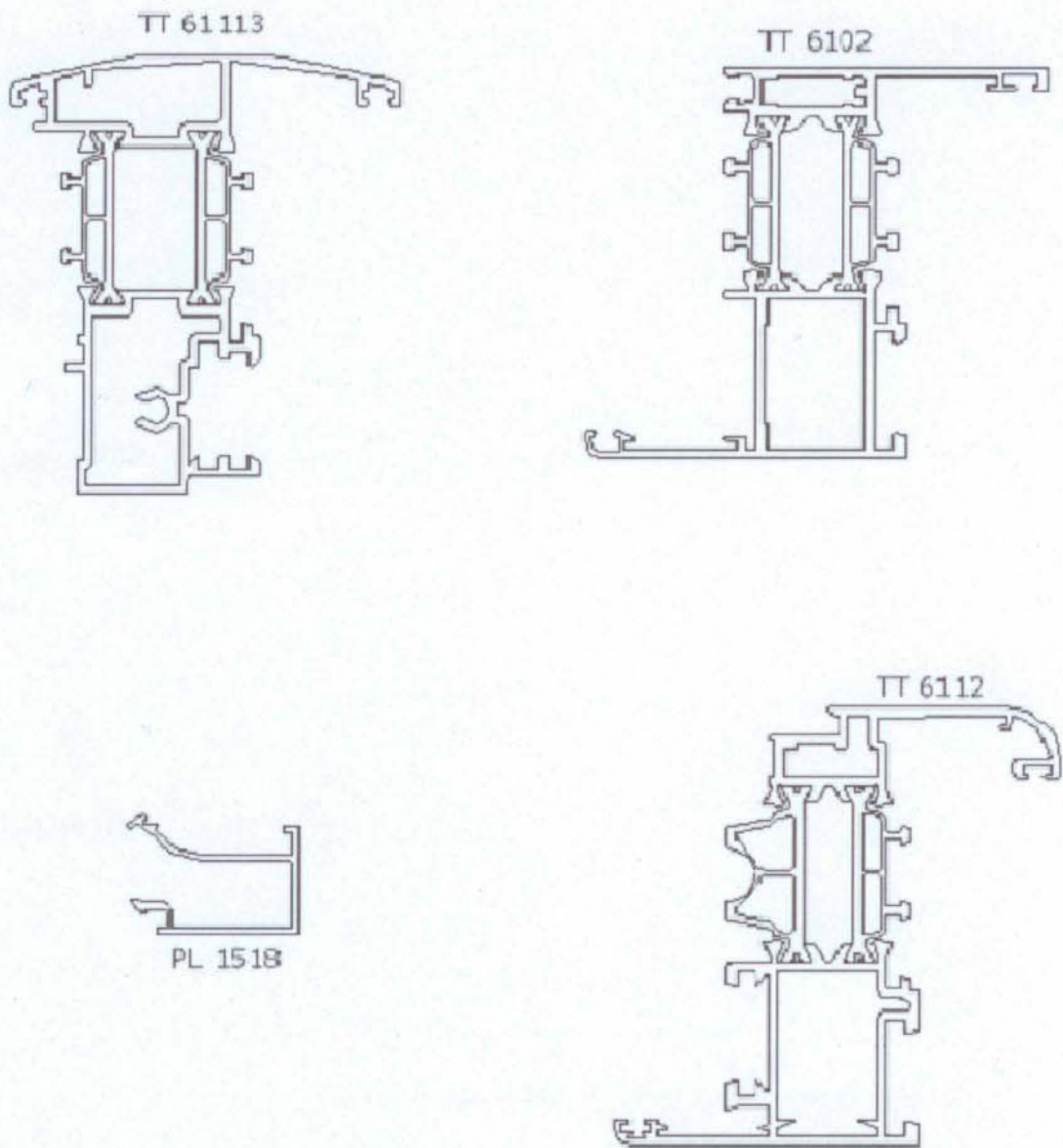
Fig.4 - Sezioni profilati.
