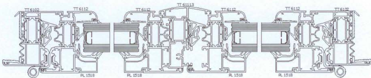
Fig.2 – Sezione orizzontale.
