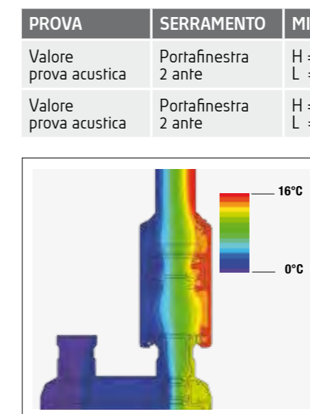
ISOTERME NODO. La figura rappresenta il comportamento delle temperature del nodo, calcolato con software specifico conforme alla norma UNI EN ISO 10077-2.
