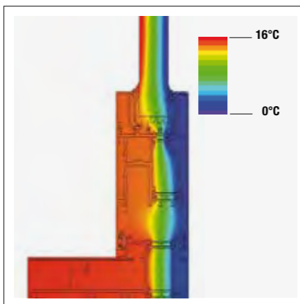
ISOTERME NODO. La figura rappresenta il comportamento delle temperature del nodo, calcolato con software specifico conforme alla norma UNI EN ISO 10077-2.
